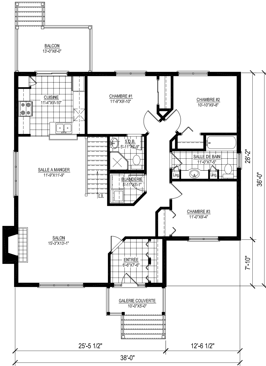
PLAN REZ-DE-CHAUSSÉE SUPERFICIE R.D.C. : 1 282 PL.CA.
