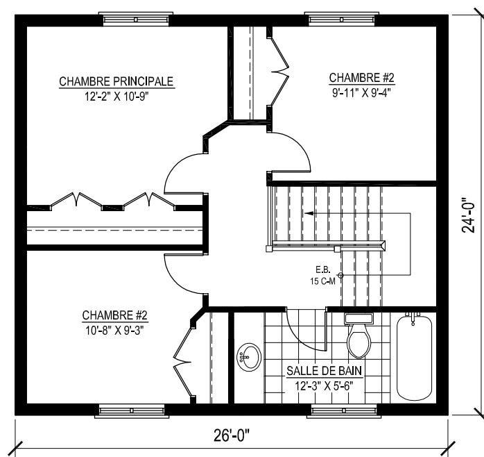
PLAN ÉTAGE #2 SUPERFICIE ÉTAGE : 624 P.I.CA.
