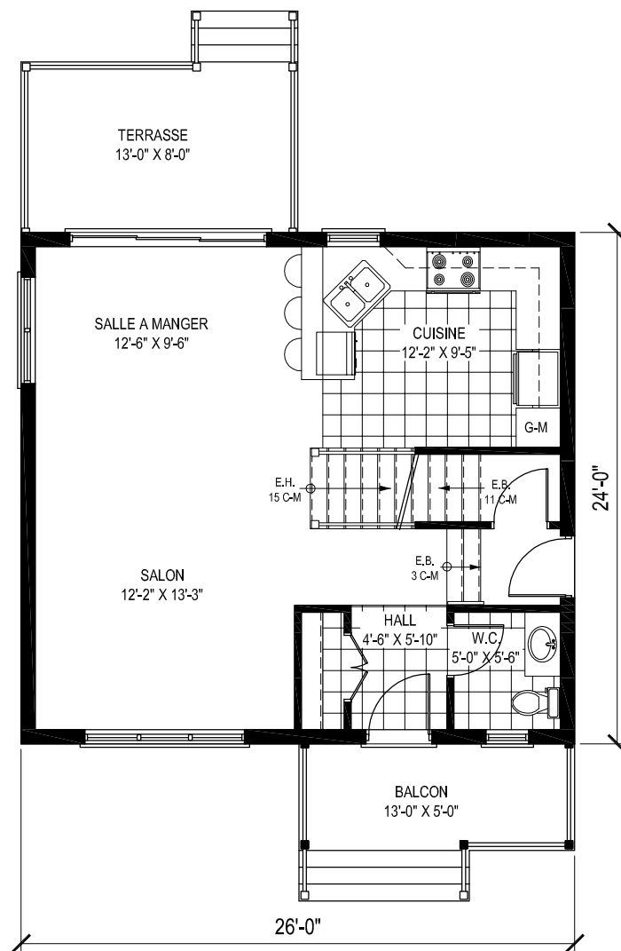
PLAN REZ-DE-CHAUSSÉE
