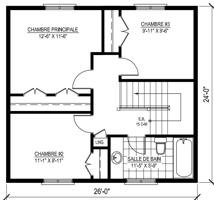
PLAN ÉTAGE #2 SUPERFICIE ÉTAGE : 624 PI.CA.
