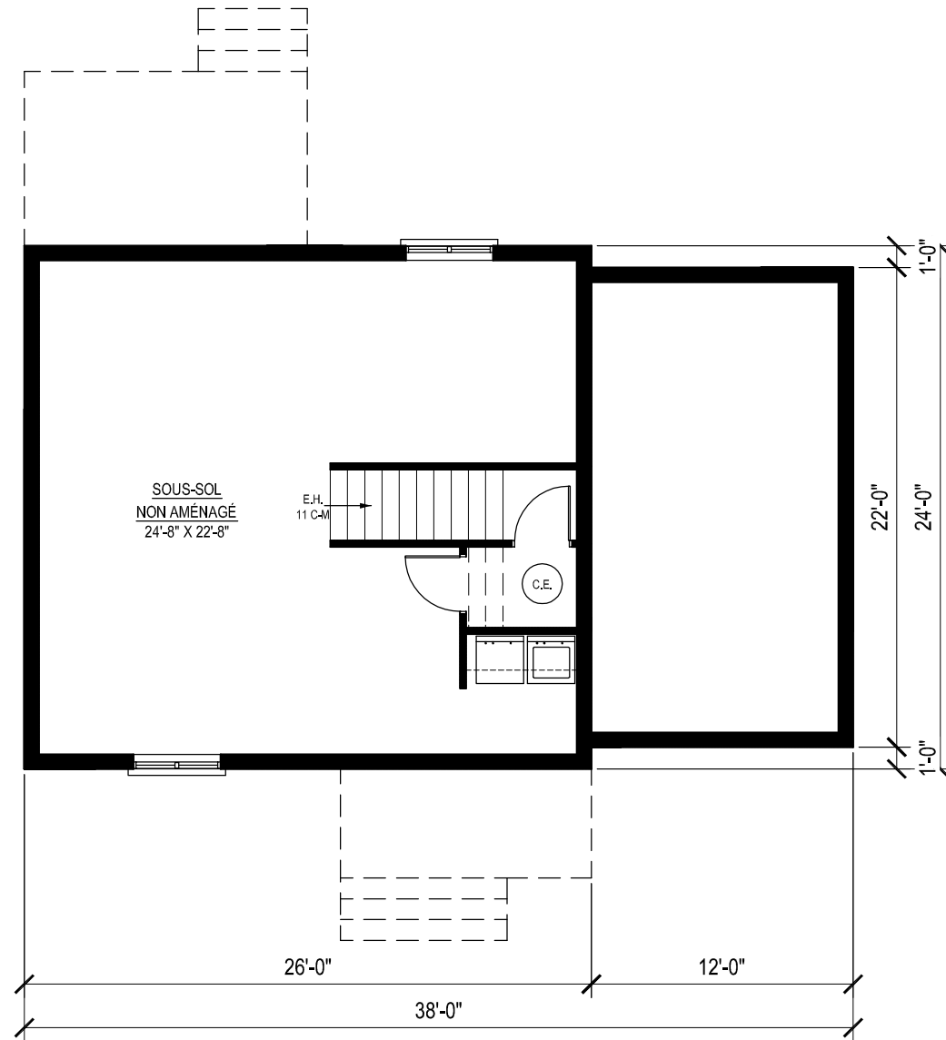
PLAN SOUS-SOL SUPERFICIE SOUS-SOL : 624 P.I.C.A.
