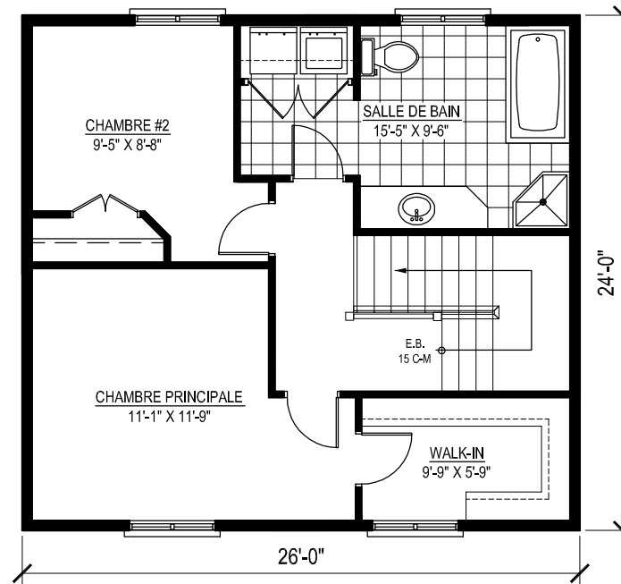
PLAN ÉTAGE #1 SUPERFICIE ÉTAGE : 624 PLCA.
