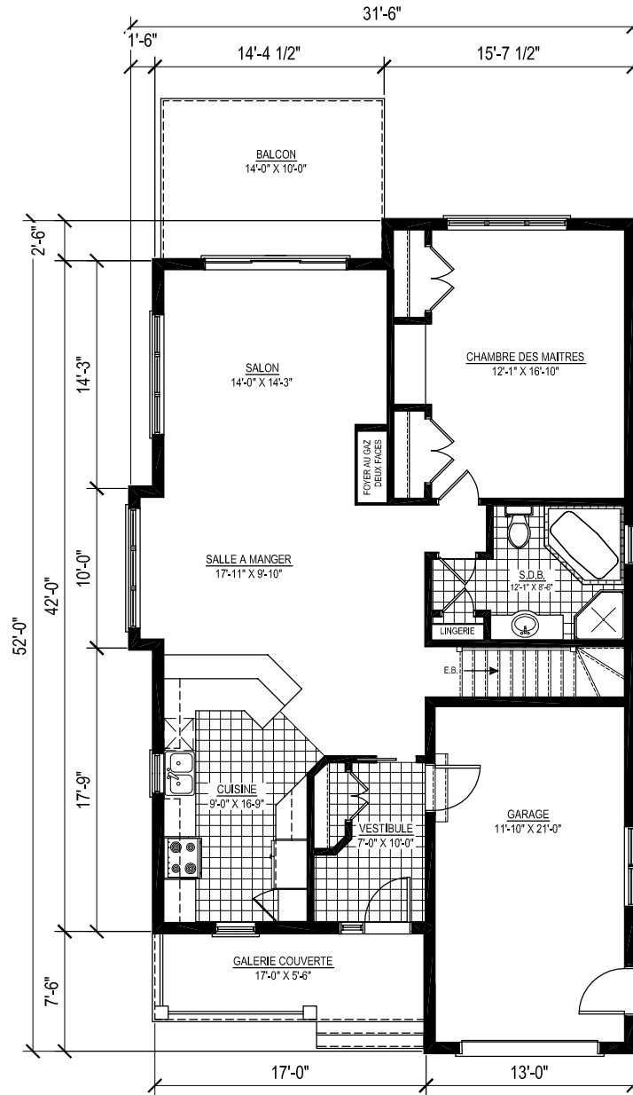
PLAN REZ-DE-CHAUSSÉE SUPERFICIE R.D.C. (PAR UNITÉ): 1 130 PI.CA. SUPERFICIE GARAGE (PAR UNITÉ): 282 PI.CA.
